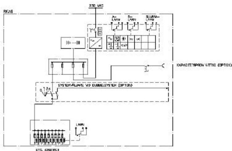
Enlinje schema med optioner
